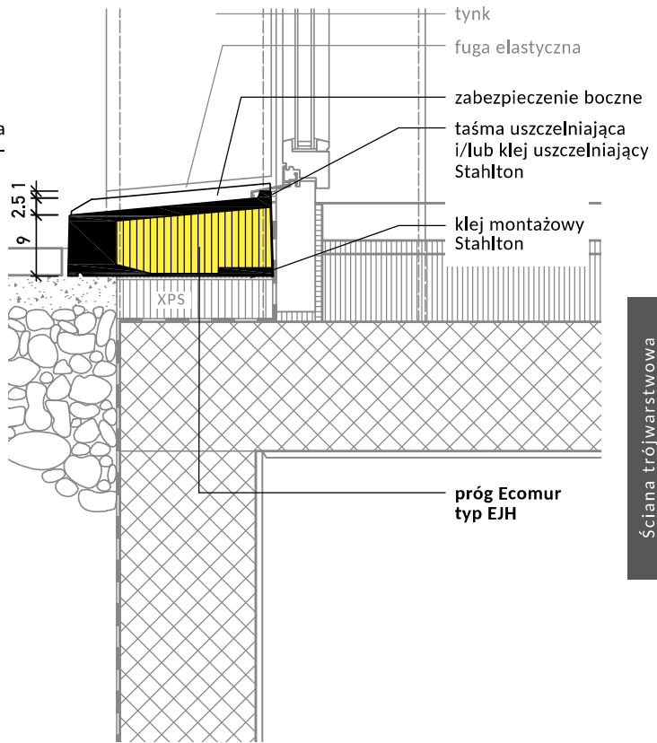
Ecomur typ EJH z zabezpieczeniem bocznym Przekrój pionowy
