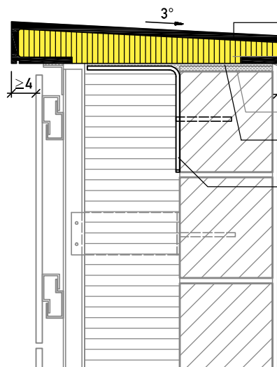
Czapa osłonowa typ EBJ z wkładką termiczną z EPS Przekrój pionowy
