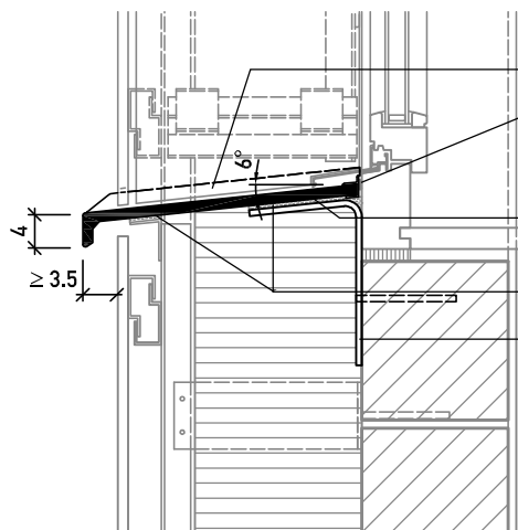
Podokiennik EL z zabezpieczeniem bocznym Przekrój pionowy
