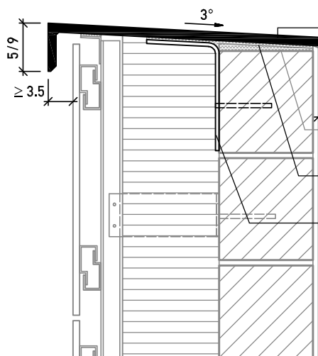
Czapa osłonowa typ EB Przekrój pionowy
