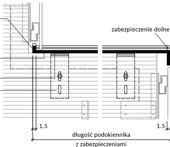
Z zabezpieczeniem górnym i dolnym Przekrój podłużny
