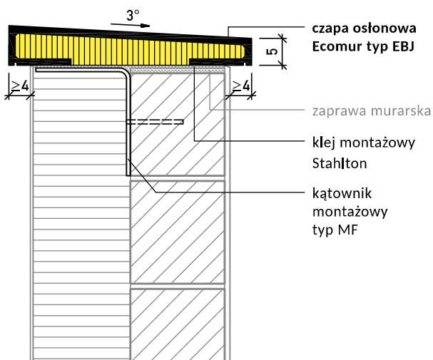
Ecomur typ EBJ (z wkładką termiczną z EPS) Przekrój pionowy
