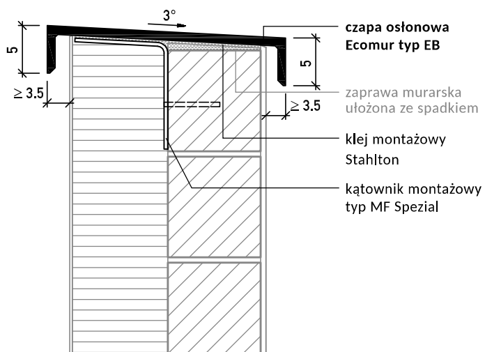
Ecomur typ EB Przekrój pionowy
