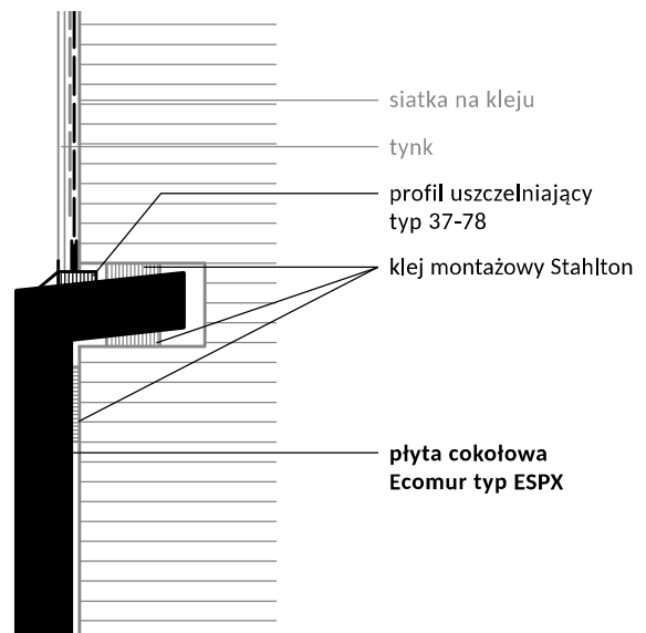
Detal połączenia B 1:2
