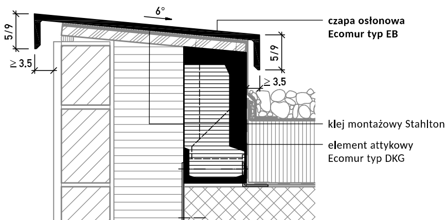
Czapa osłonowa Ecomur typ EB Przekrój pionowy
