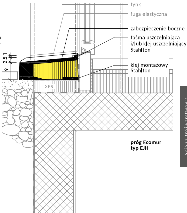
Ecomur typ EJH z zabezpieczeniem bocznym Przekrój pionowy
