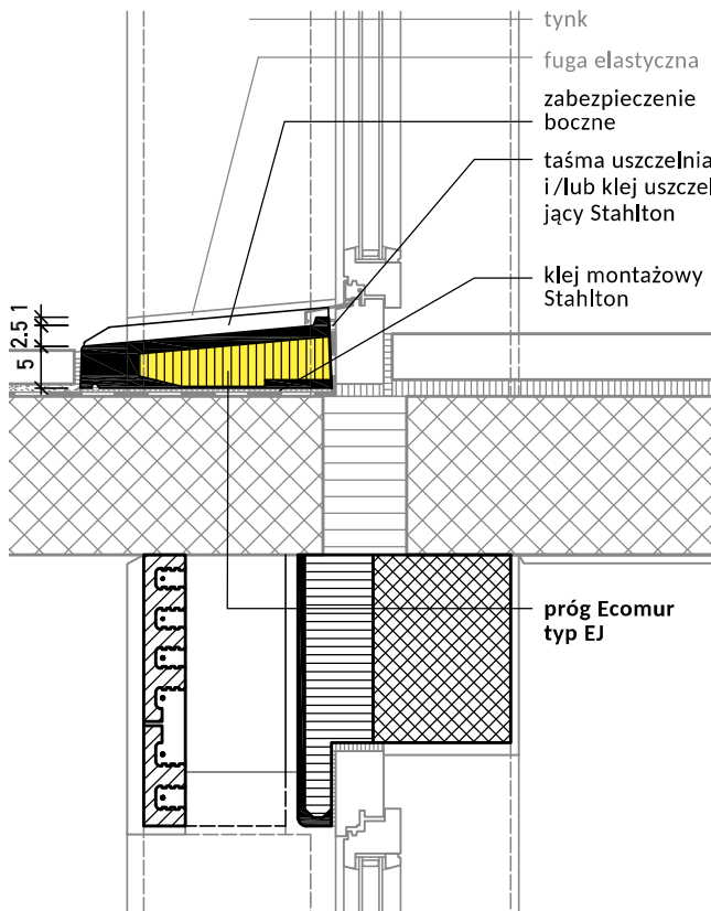
Ecomur typ EJ z zabezpieczeniem bocznym Przekrój pionowy
